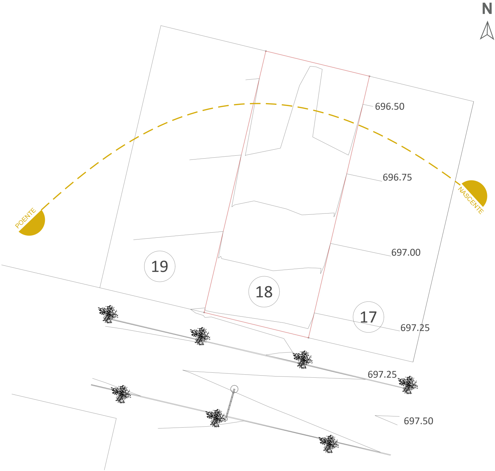
LEVANTAMENTO PLANIALTIMÉTRICO S/ ESCALA
