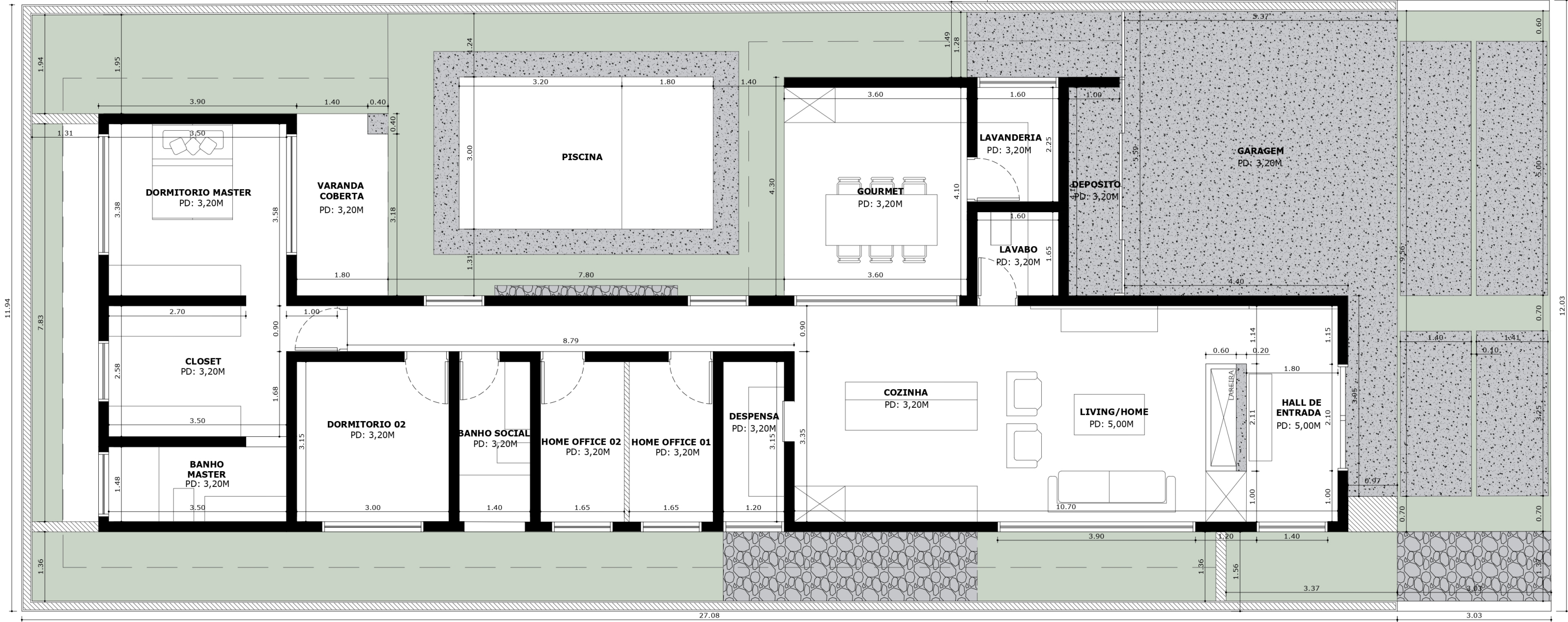
PLANTA BAIXA S/ ESCALA
